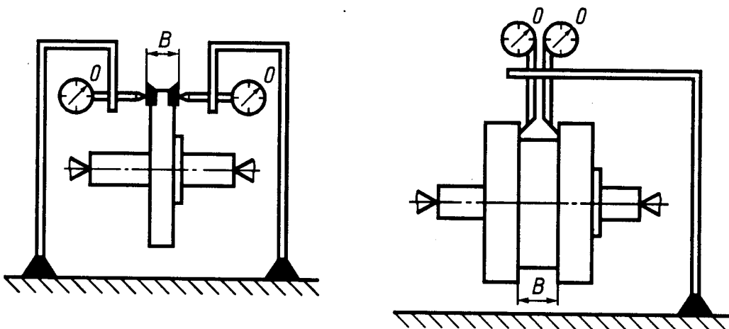
Схема измерения ширины фрез
