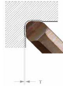
Пример обработки канавки
