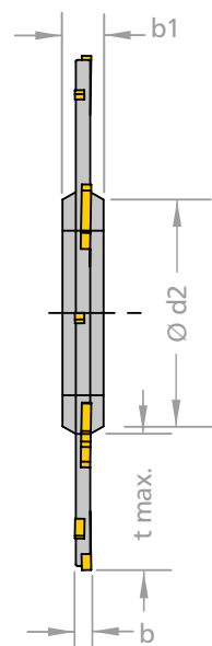
Посадочное отверстие со шпонкой по DIN 138
